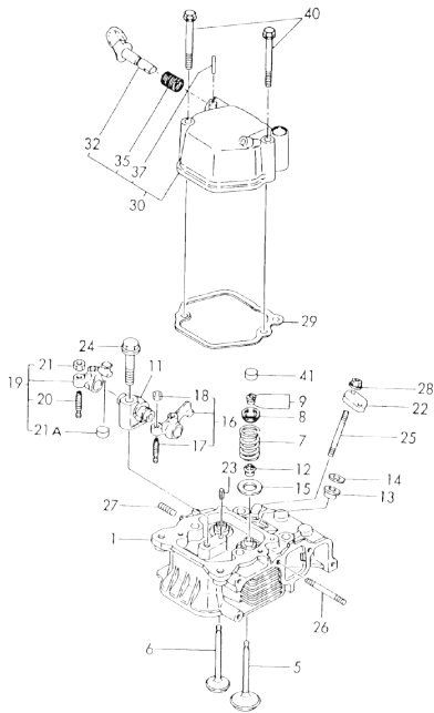
Fig. 12 シリンダヘッド & ホンネット CYLINDER HEAD & BONNET
