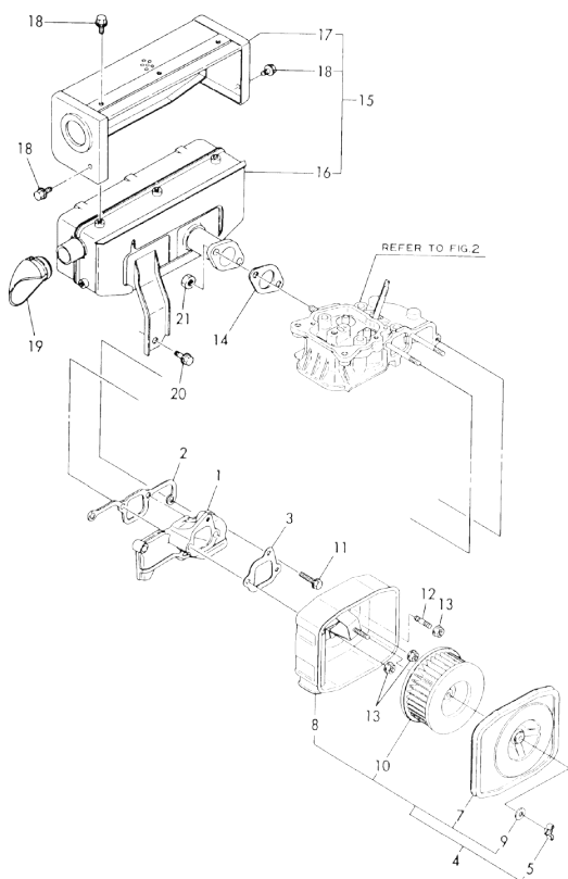
Fig. 3 エアクリーナ&マフラ AIR CLEANER & MUFFLER
