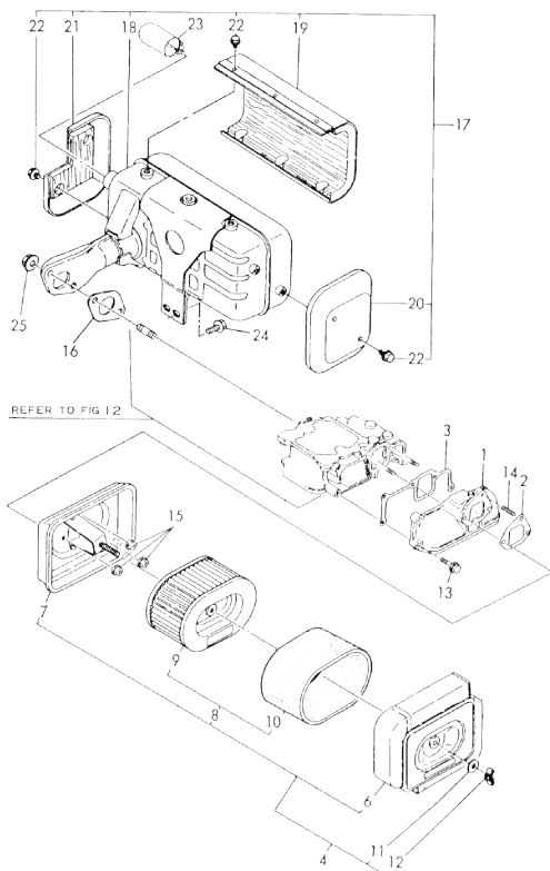
Fig. 13 エアクリーナ&マフラ AIR CLEANER & MUFFLER
